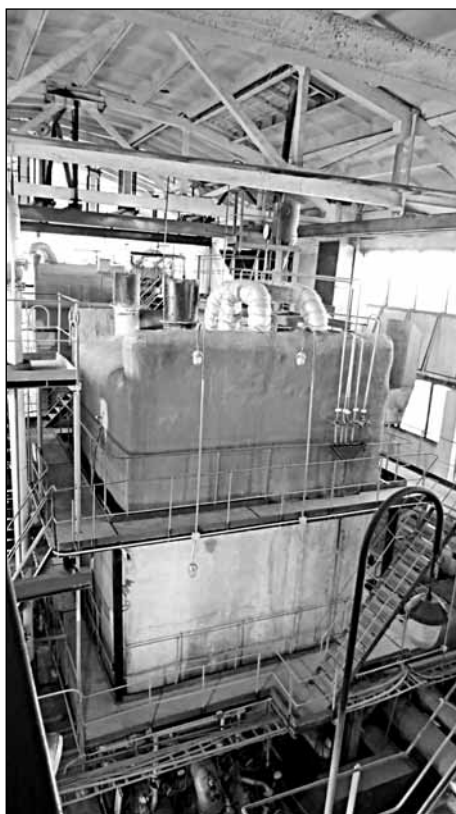
Левобережная котельная. Котёл 35МВт 1978 года выпуска
